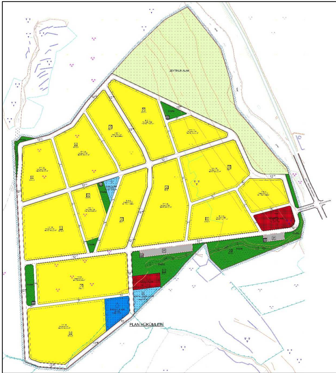
Harita 10-1: 1/1000 Ölçekli Uygulama İmar Planı
